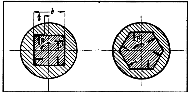
Fig. 3—Square type
